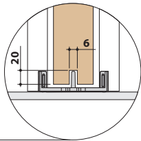
PARA 2 PORTAS (dimensões em mm)
