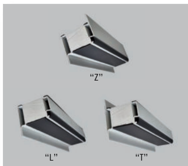
Aro tubular com 3 versões de perfil: "Z", "L" e "T".
