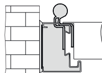
Com aro tubular ignífugo (extra)
