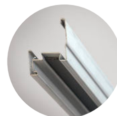
Perfil do aro com guarnição intumescente
